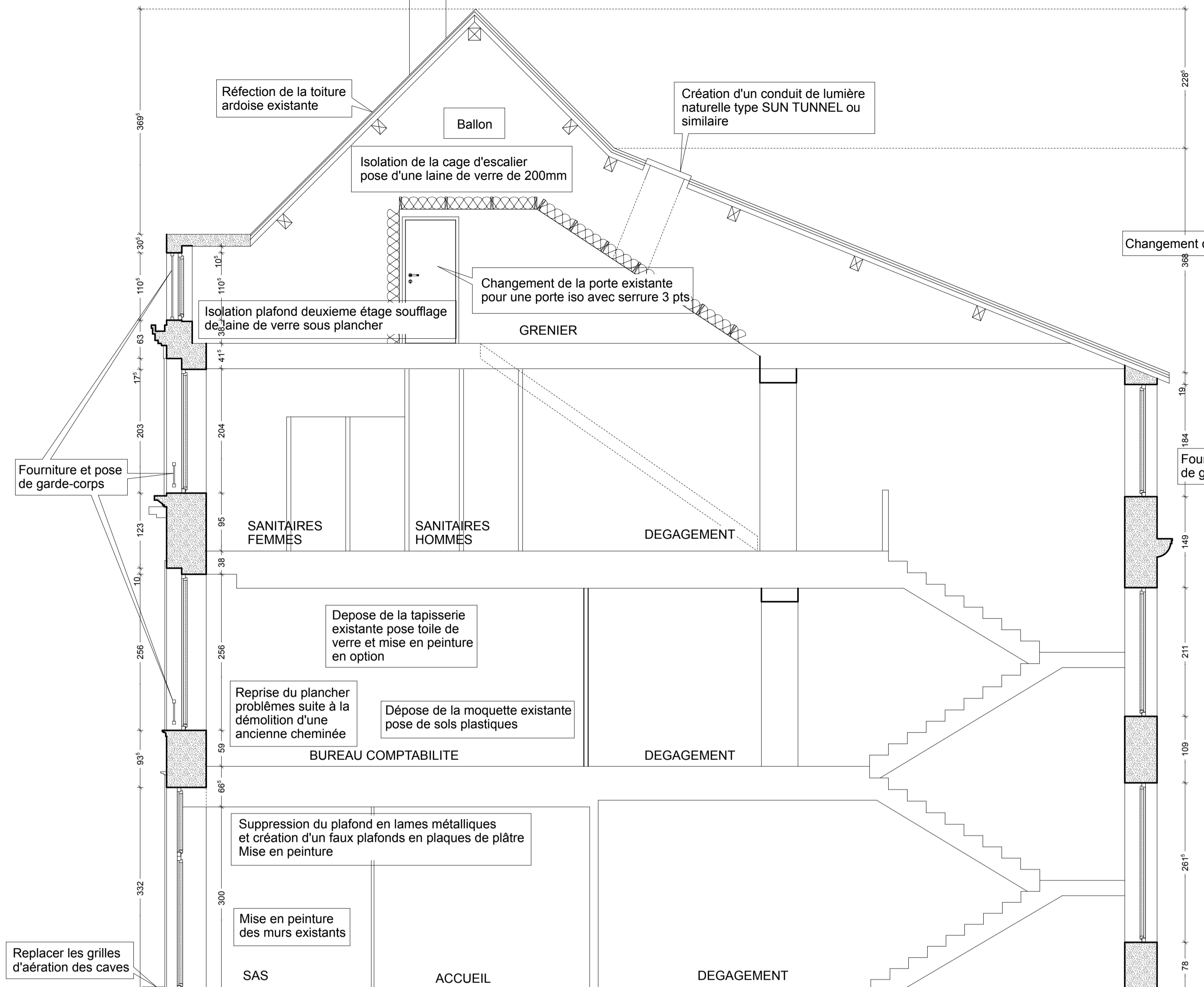
CAVES NON RELEVÉES COUPE BB PROJET
