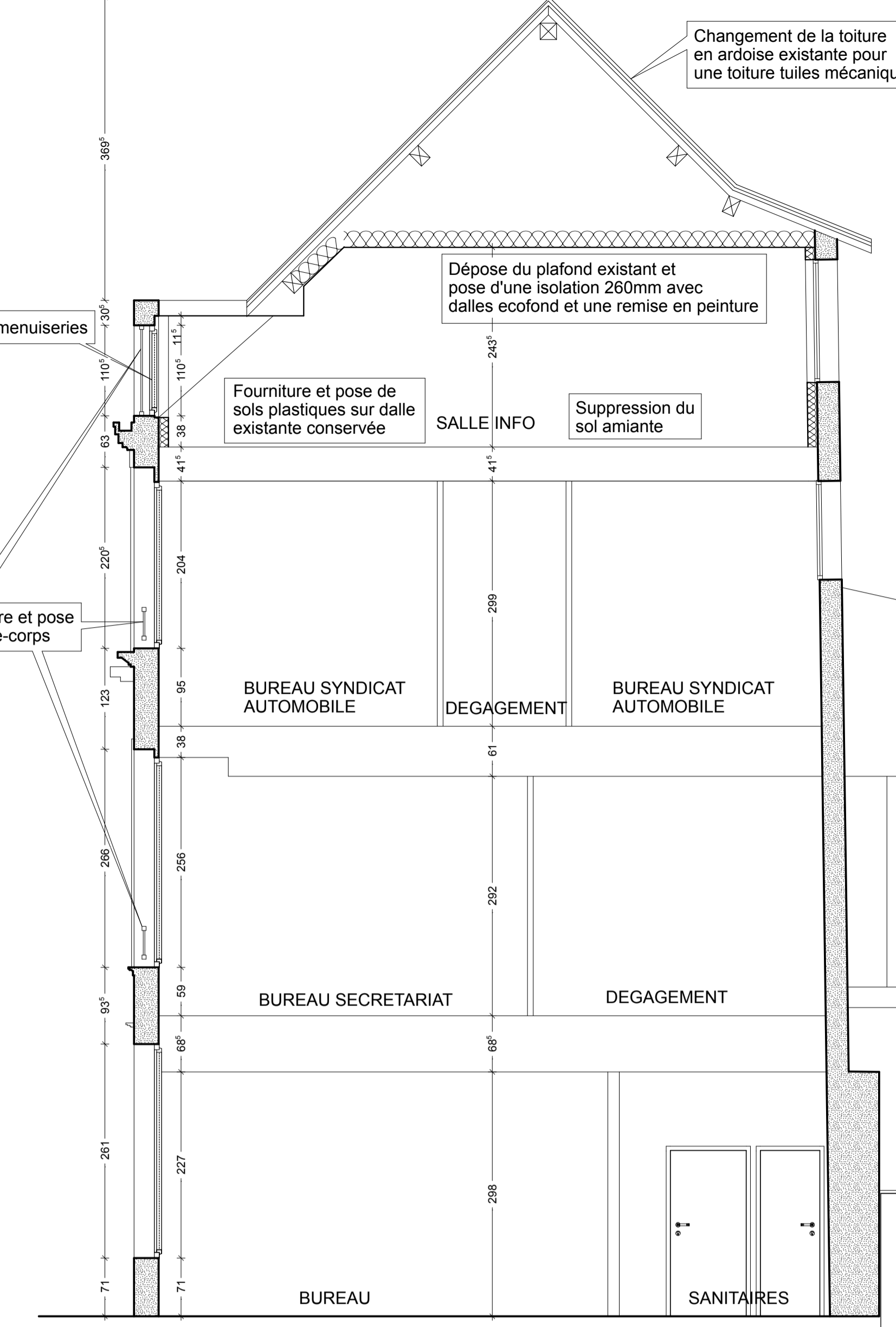
COUPE AA PROJET
